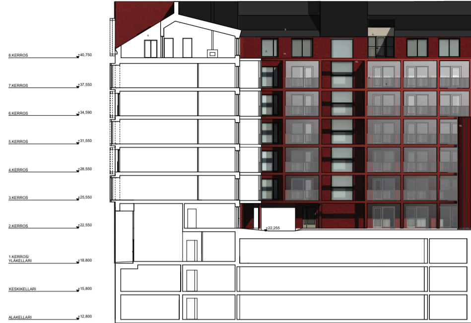
LEIKKAUS JA PIHAJULKISIVU LÄNTEEN 1:400
