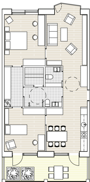
ASUNTO 3H+K(T)+S 89,5 m 2 VAIHTOEHTO 1
