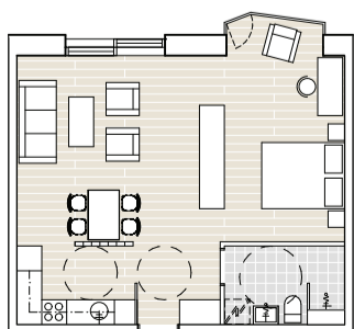
ASUNTO 2H+KT 51,0 m 2 VAIHTOEHTO 1
