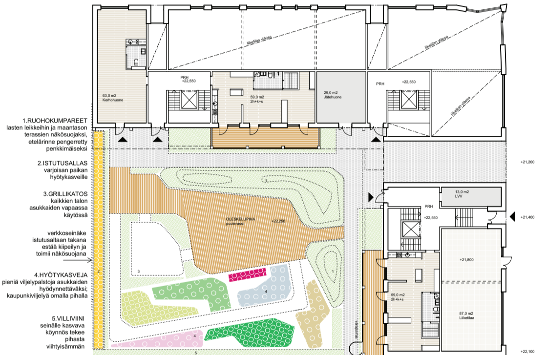
2. KERROS 1:400
